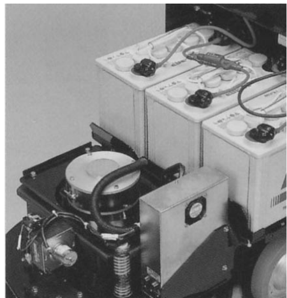
写真2 DE-501 型搭載電池外観
